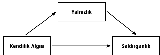
Şekil 1: Path Diyagramı
